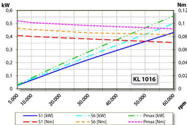
Leistungsdiagramm Spindelträgerkühlung
