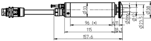
寸法図
