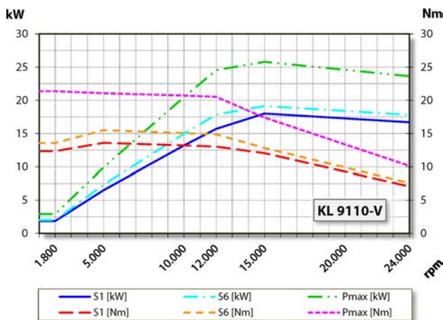
Diagram výkonu
