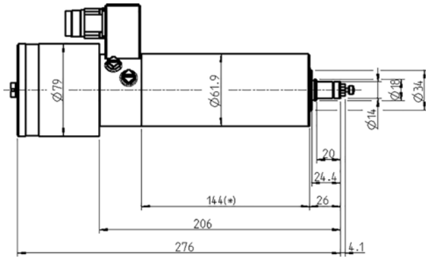
尺寸
